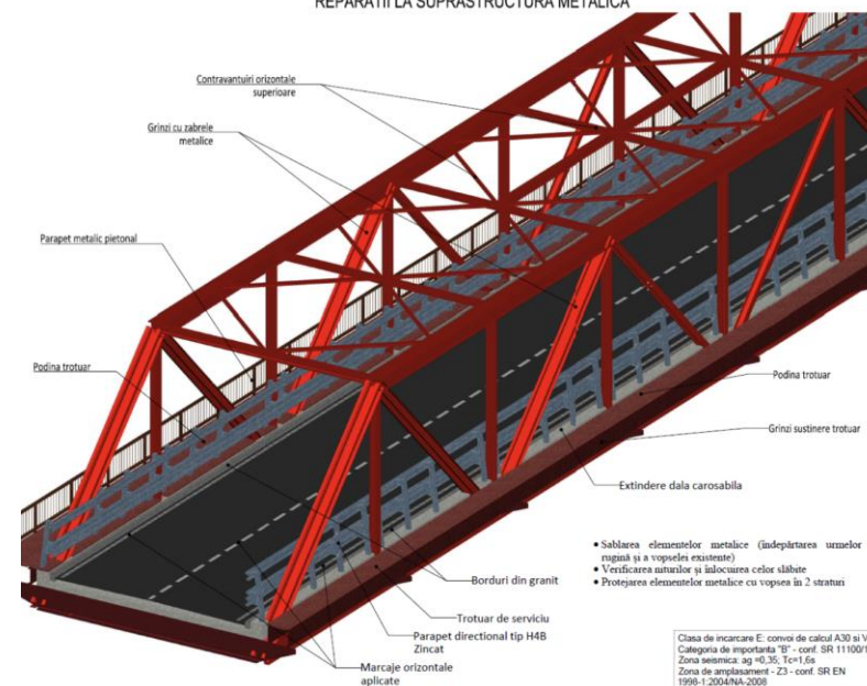
REPARATII LA SUPRASTRUCTURA METALICA
